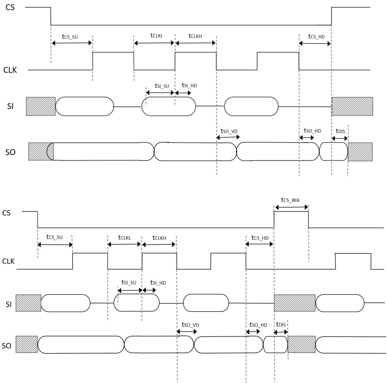
图 3-3 SPI 时序图
